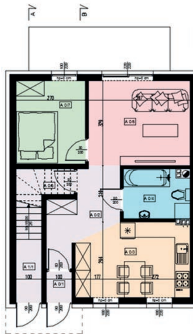
Projekt parterowego mieszkania o pow. 49 m 2 w budynku dwulokalowym
