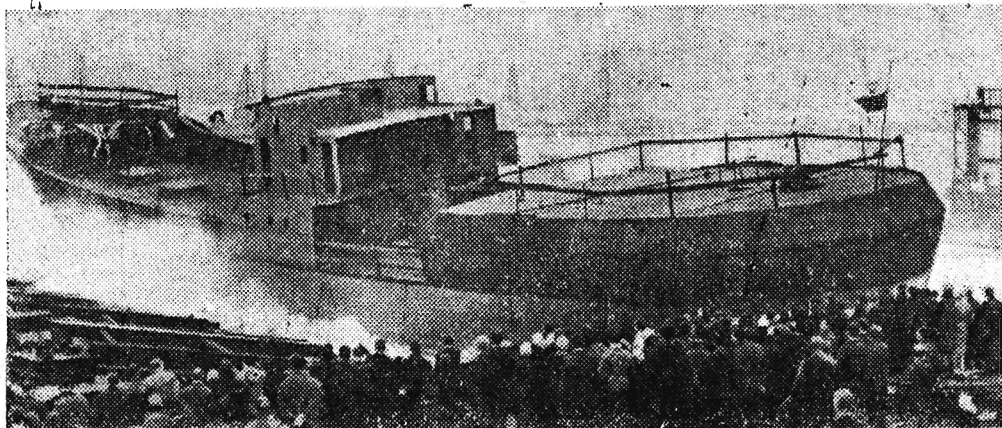
W stoczni im. Komuny Paryskiej w Gdyni wodowano pierwszą jednostkę rybacką z serii nowoczesnych motorowych trawlerów. Patronat nad budową tej serii objęła młodzież z ZMS. Na zdjęciu: Moment bocznego wodowania. CAF — fot. Błażewicz
