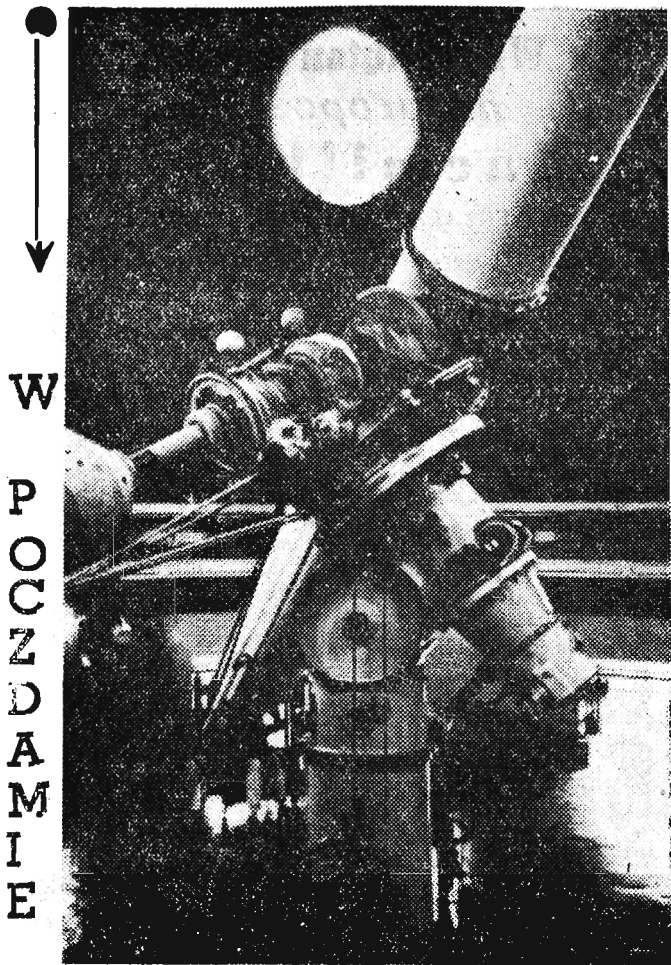
W Poczdamie — Dabelsberg k/Berlina znajduje się Obserwatorium Astronomiczne Niemieckiej Akademii Nauk. Na zdjęciu: Duży refraktor Zeissa, Ogniskowa 10,5 m, otwór obiektywu 65 cm. Fot — CAP
