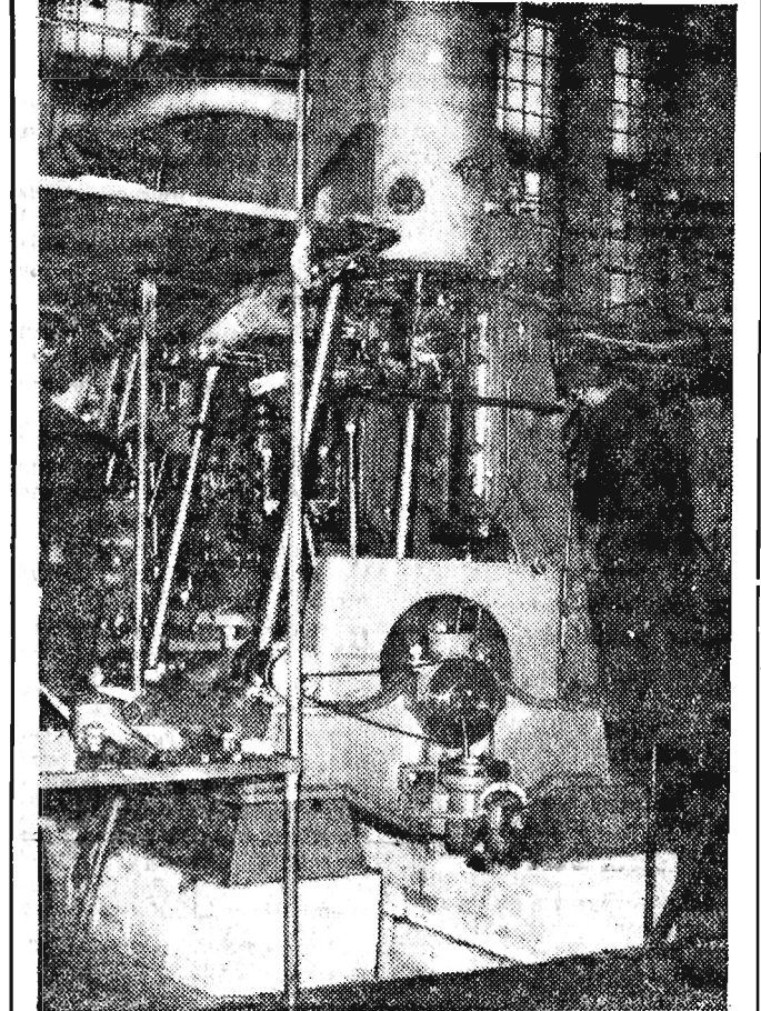
W zakładach H. Cegielskiego w Poznaniu rozpoczęto w br. seryjną produkcję maszyn okrętowych o mocy 300 KM. Na zdjęciu: Fragment montażu maszyny okrętowej. CAF — fot. Kondracki
