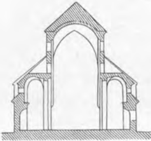
Fig. 19. Durchschnitt von Heisterbach.
