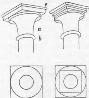
Fig. 29. Kelchkapitäl.
