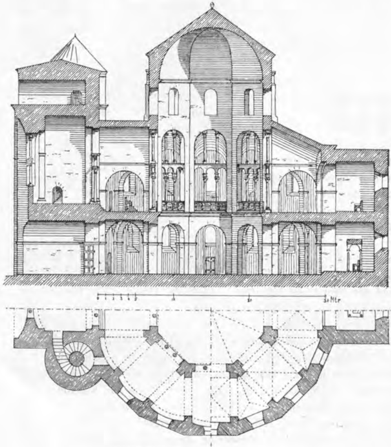
Fig. 10. Plan und Durchschnitt des Münsters zu Aachen.
