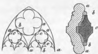
Fig. 74. Pfostenwerk.
