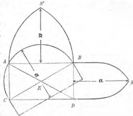
Fig. 55. Gewölbeschema.
