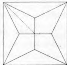
Fig. 59. Netzwölbe.
