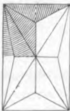
Fig. 57. Sterngewölbe.
