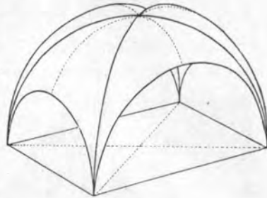
Fig. 38. Das überhöhte, busige Kreuzgewölbe.
