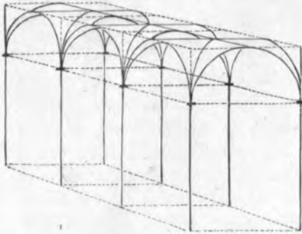
Fig. 37. Kreuzgewölbe (Geripp)
