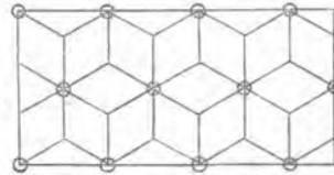
Fig. 60. Netzgewölbe.
