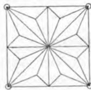
Fig. 58. Sterngewölbe.
